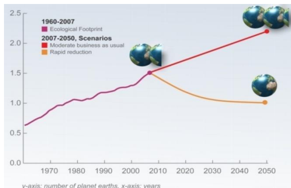
Slika 4. Prikaz zagađenja planete zemlje do 2007. godine i scenarija razvoja događaja do 2050. godine
