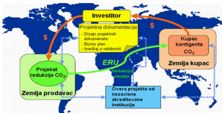
Slika 6. Model funkcionisanja trgovine sa \text{CO}_2 u svetu [7]
