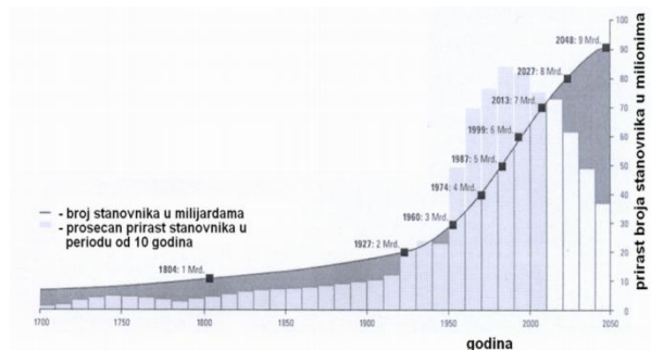
Slika 2. Porast broja stanovnika na zemlji od 1700. do 2007. godine i prognoza do 2050. godine
